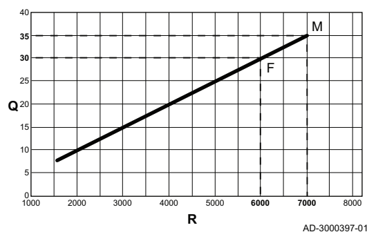
Abb.51 Wärmebelastung EMC-M 34/39MI Plus
