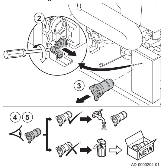
Abb.61 Reinigen des Wasserfilters
