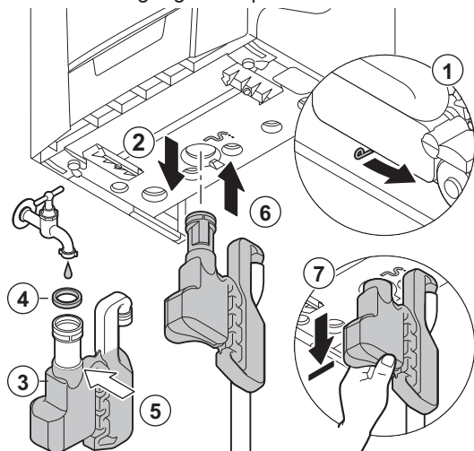
Abb.56 Reinigung des Siphons
