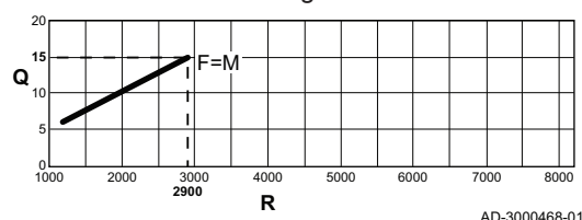
Abb.48 Wärmebelastung EMC-M 25 Plus
