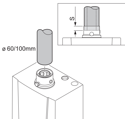
Abb.24 Anschluss des Abgasstutzens und der Luftzuführung
