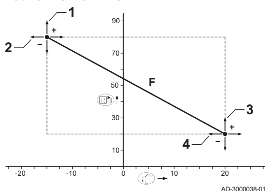
Abb.29 Heizkennlinie
