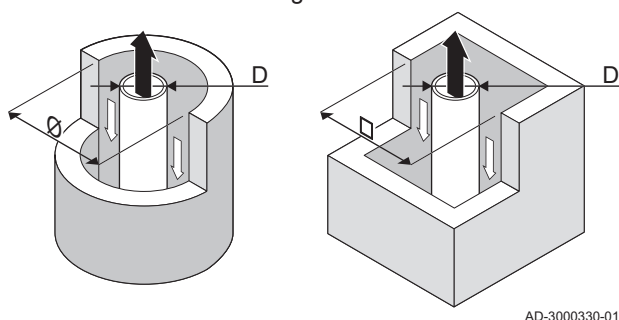
Abb.23 Mindestabmessungen des Schachts oder Kanals
