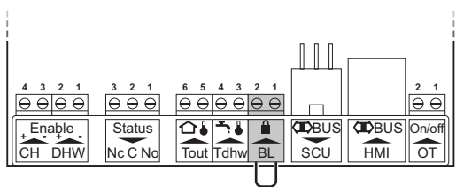
Abb.35 Sperreingang
