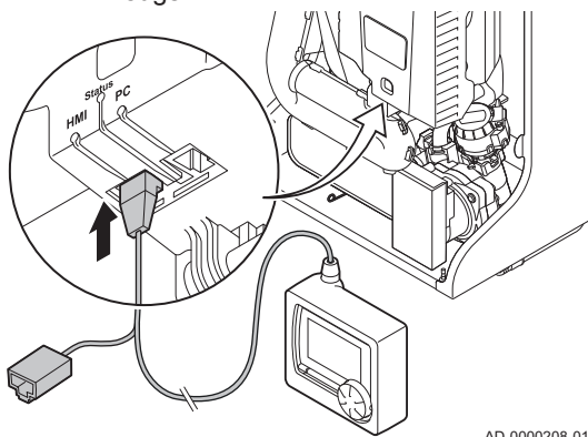
Abb.37 Anschließen eines Wartungswerkzeugs
