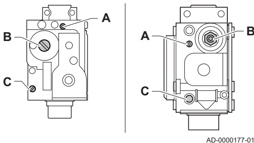
Abb.42 Prüfüffnungen der Gasventilbaugruppe
