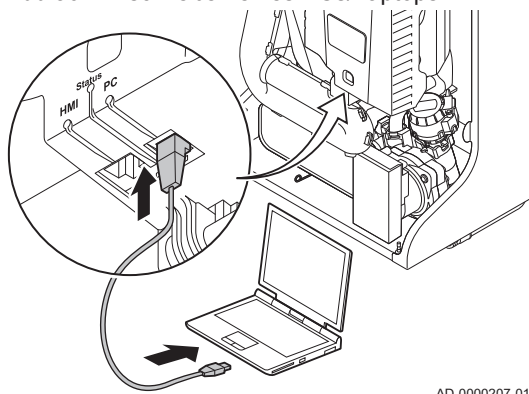
Abb.36 Anschließen eines PCs/Laptops
