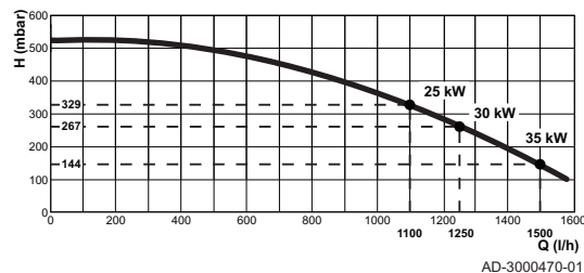
Abb.5 EMC-M 35 Plus - 34/39MI Plus
