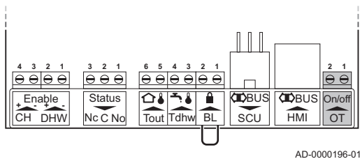
Abb.26 Anschluss eines modulierenden Thermostats
