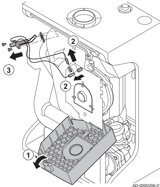
Abb.58 Austausch der Ionisations- bzw. Zündelektrode
