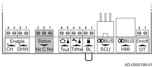
Abb.33 Betriebssignal und Fehlersignal
