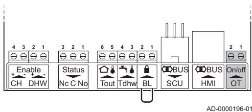
Abb.27 Anschluss des Ein/Aus-Thermostats
