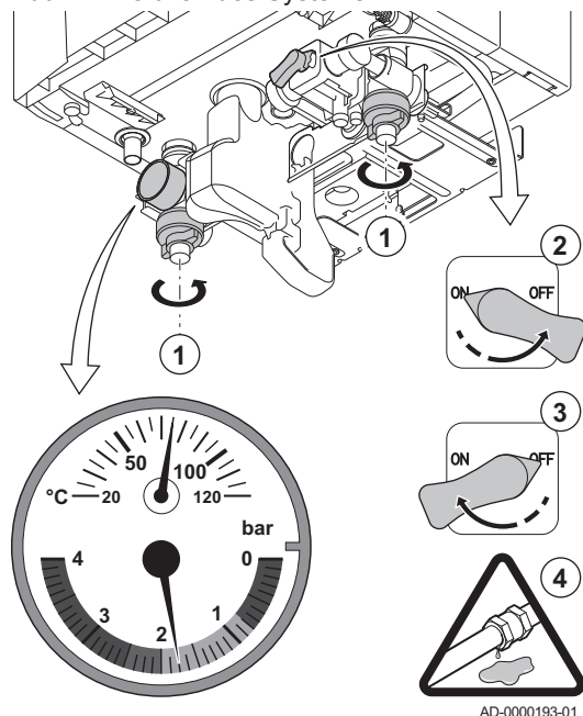
Abb.41 Befüllen des Systems
