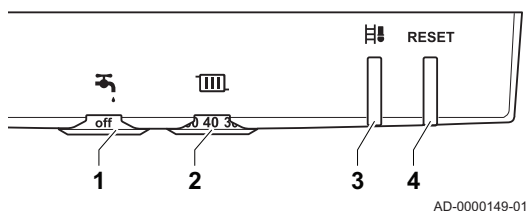
Abb.65 Kesselschaltfeld
