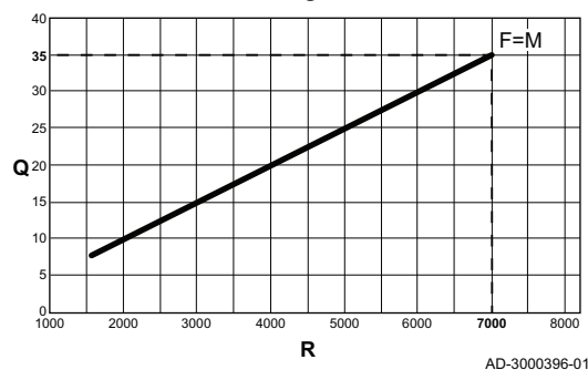
Abb.51 Wärmebelastung EMC-M 34/39MI Plus
