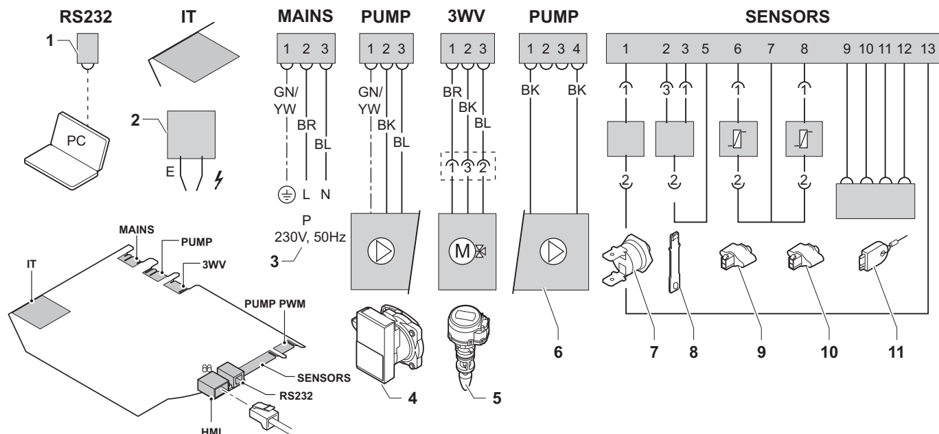
Abb.2 Elektrischer Schaltplan
