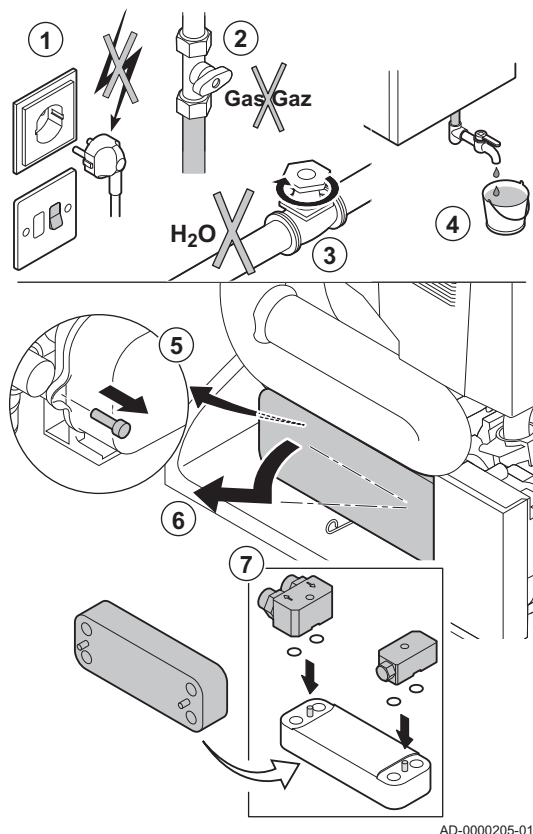
Abb.60 Reinigen des Plattenwärmetauschers
