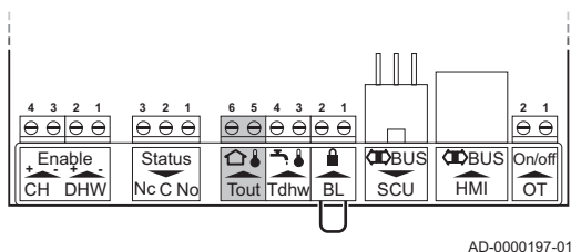
Abb.28 Anschluss eines Außenfühlers
