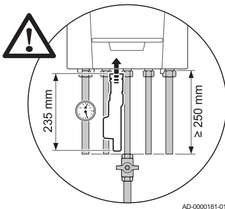
Abb.15 Platz für Einbauten unter dem Kessel
