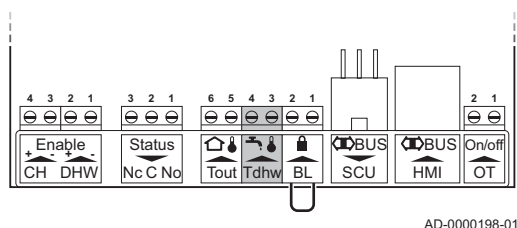
Abb.32 Anschließen des Fühlers/Thermostats für den Warmwasserbereiter
