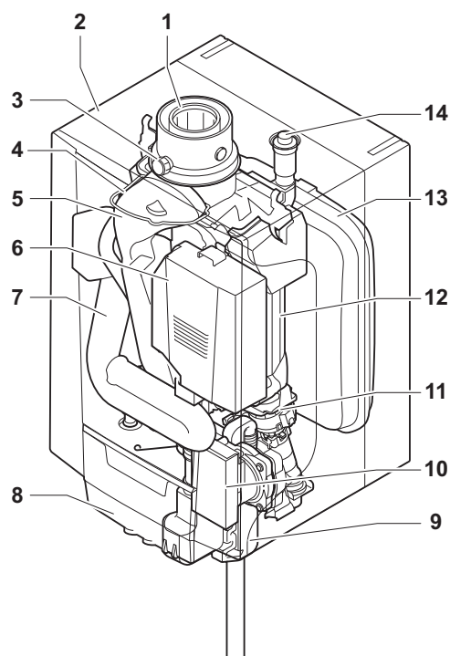
Abb.8 EMC-M 15 Plus - 25 Plus - 35 Plus
