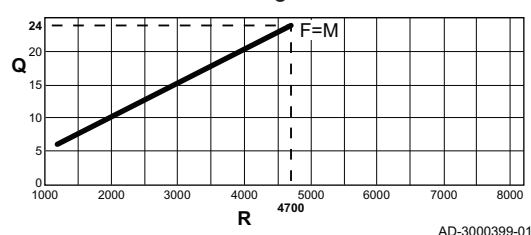
Abb.48 Wärmebelastung EMC-M 25 Plus
