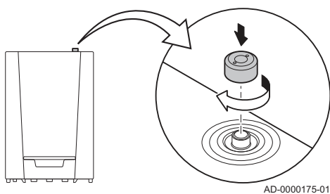
Abb.20 Automatischer Schnellentlüfter
