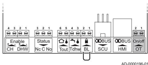
Abb.30 Anschluss des Frostschutzthermostats
