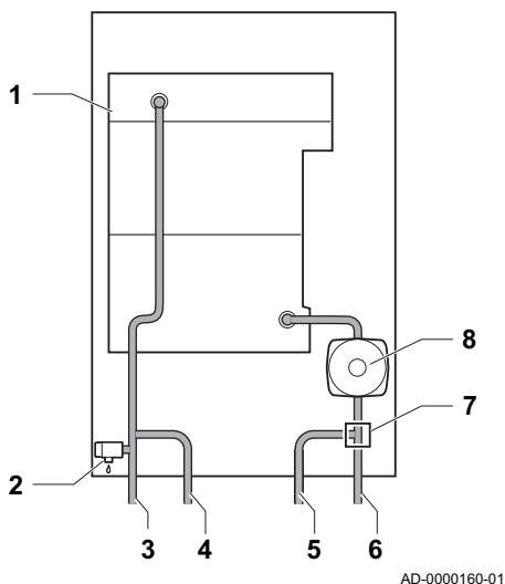
Abb.6 EMC-M 15 Plus - 25 Plus - 35 Plus
