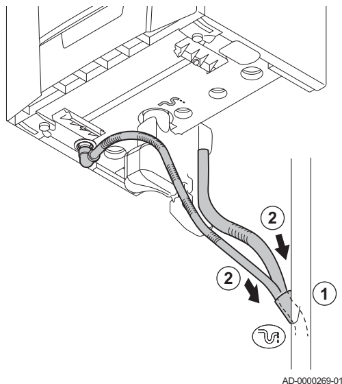
Abb.19 Anschluss der Kondensatablaufeitung
