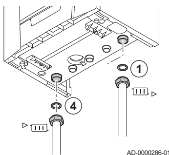
Abb.16 Anschluss des Heizkreises
