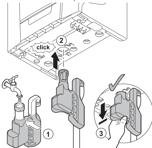
Abb.39 Befüllen des Siphons
