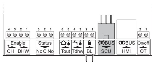
Abb.38 Anschlüsse für optionale Leiterplatten
