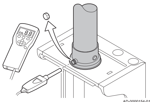
Abb.43 Prüfüffnung für Abgas
