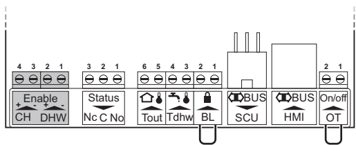
Abb.34 Anschließen des Ein/Aus-Kontakts (Aktivieren)
