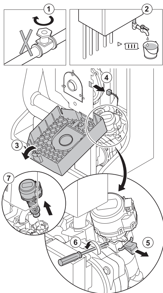
Abb.59 Auswechseln des Dreiwegeventils
