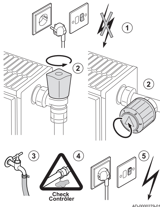
Abb.40 Befüllen des Systems
