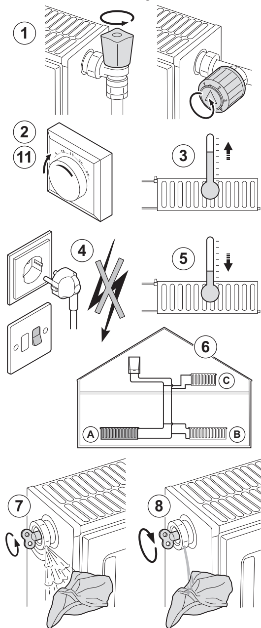
Abb.64 Entlüften der Anlage
