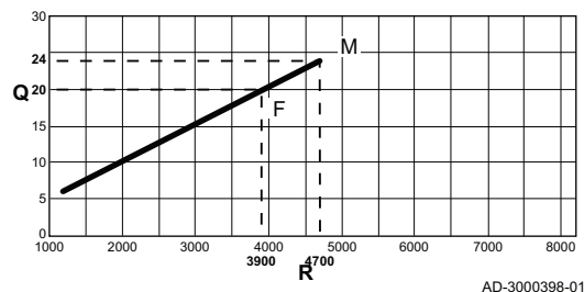
Abb.50 Wärmebelastung EMC-M 35 Plus
