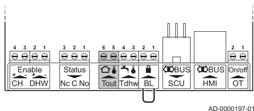
Abb.31 Anschluss eines Außenfühlers
