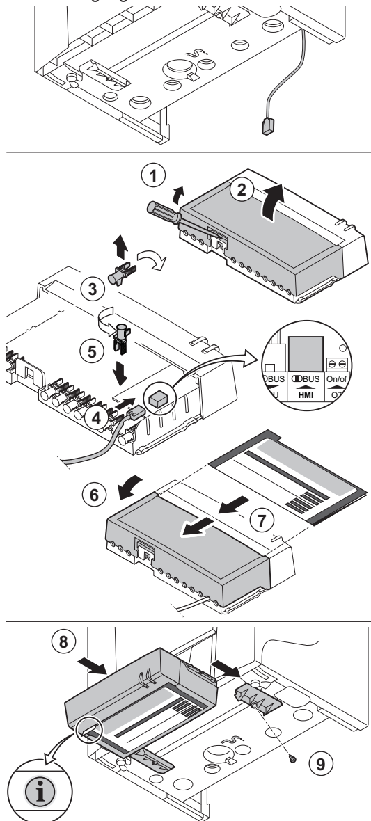
Abb.25 Zugang zu den Anschlüssen
