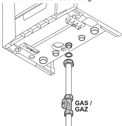
Abb.21 Anschluss der Gasleitung
