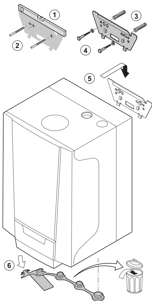
Abb.14 Montage des Heizkessels
